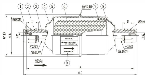
螺口 Thread
